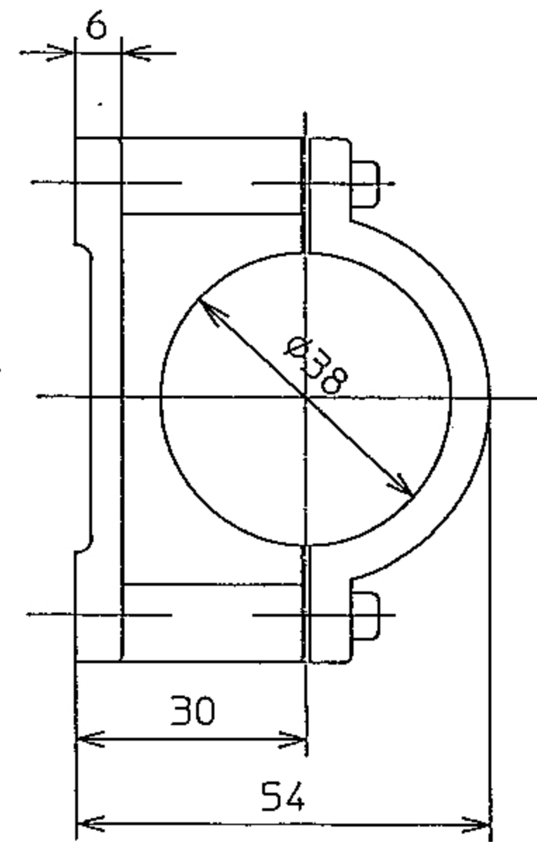
取付金具 Type 2047
