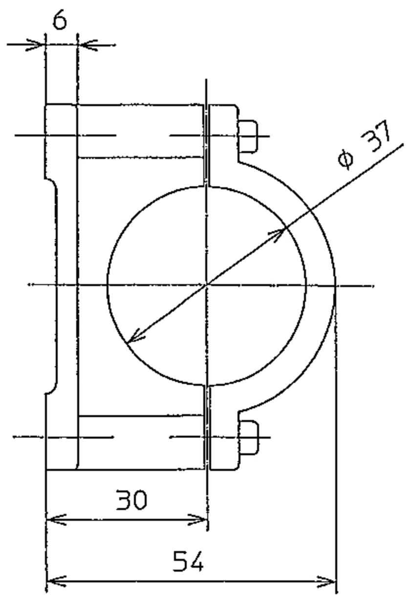
取付金具 Type 2046
