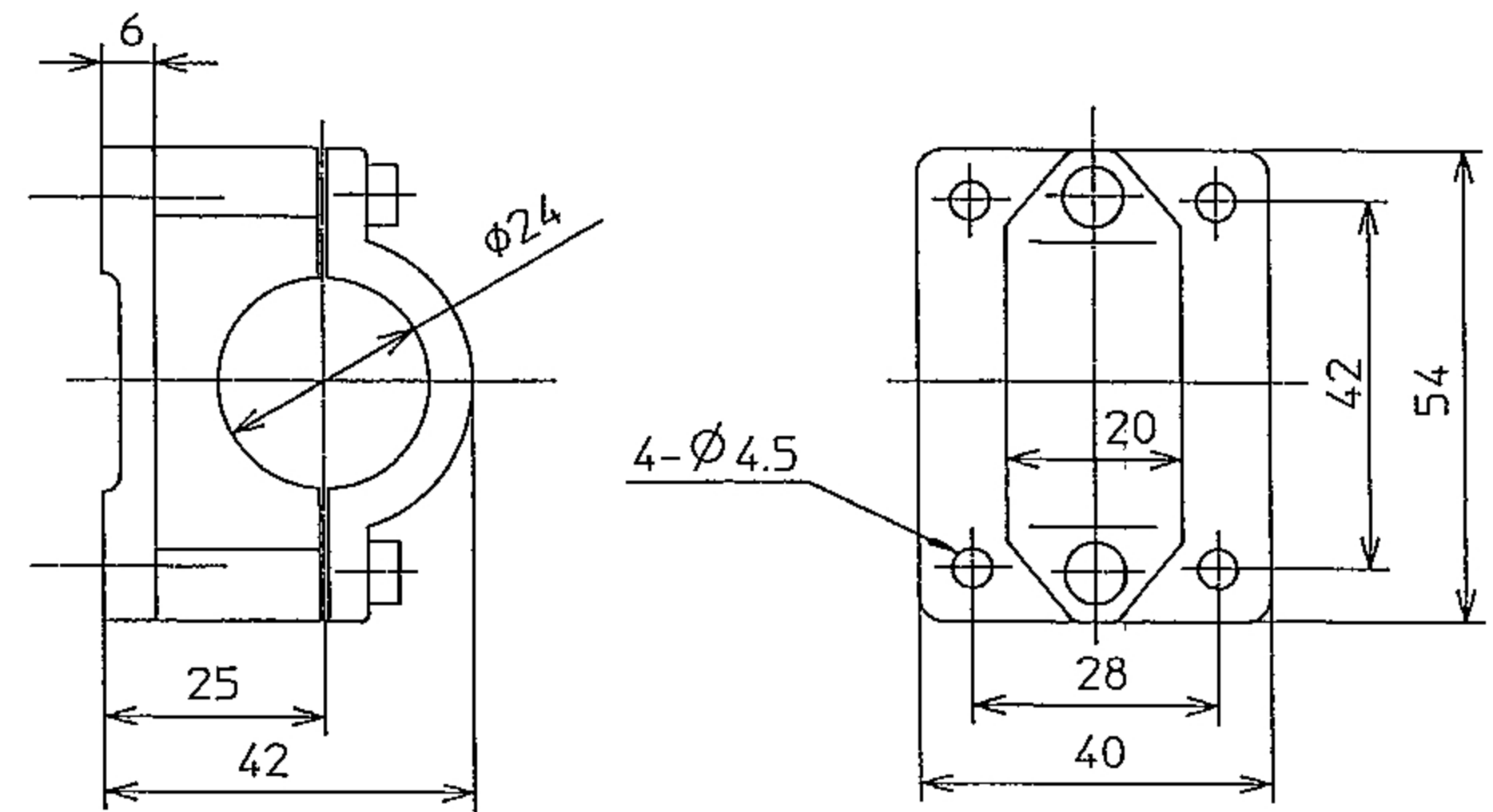
取付金具 Type 2044
