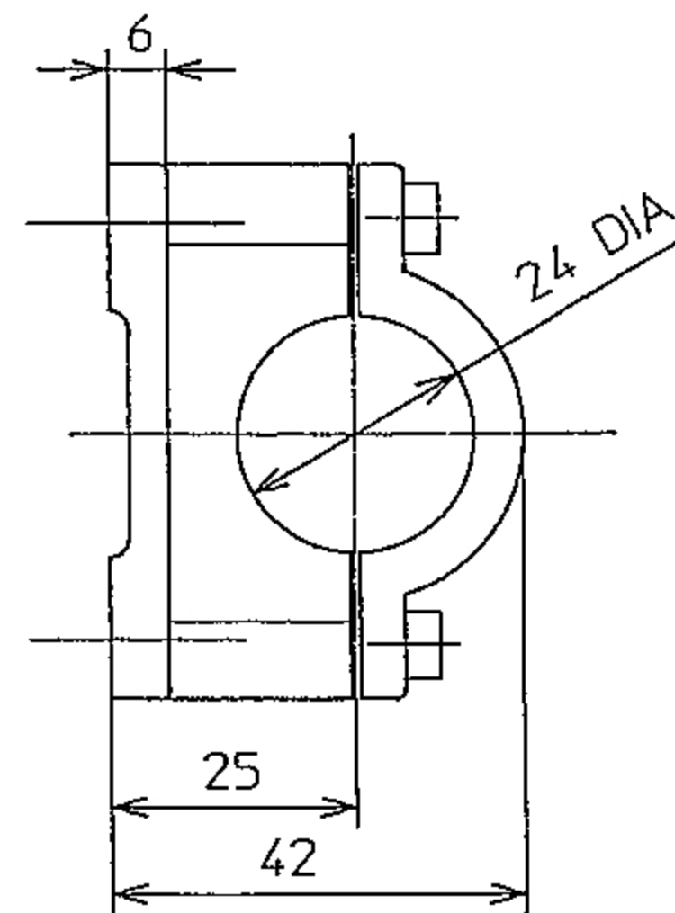
取付金具 Type 2044
