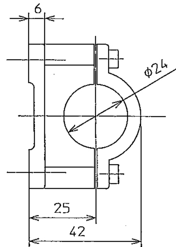
取付金具 Type 2044
