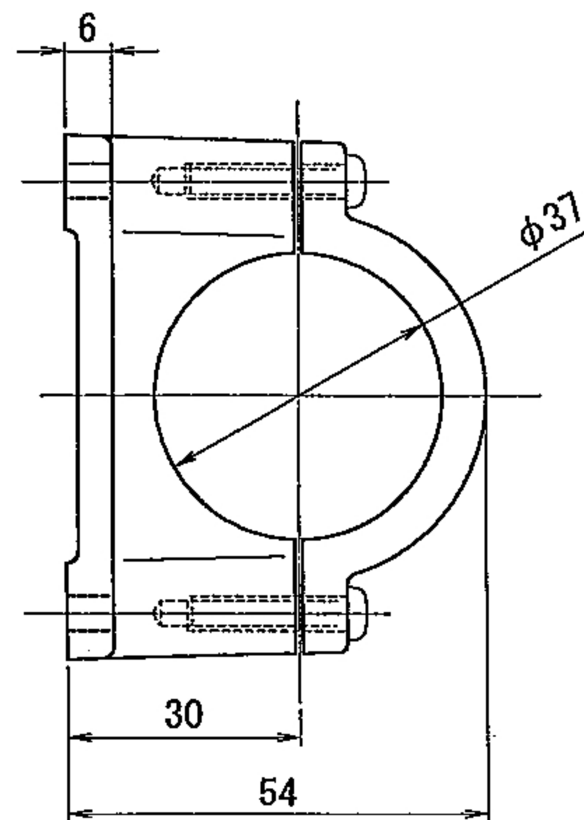
取付金具 Type 2046
