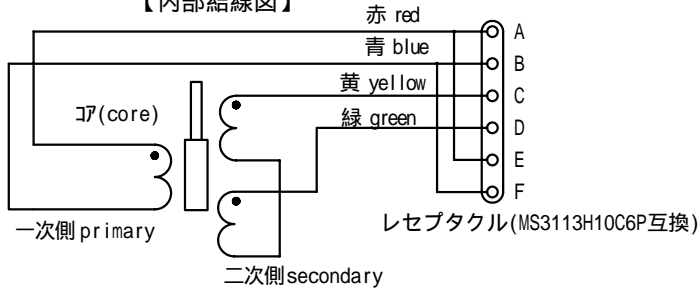
【内部結線図】
